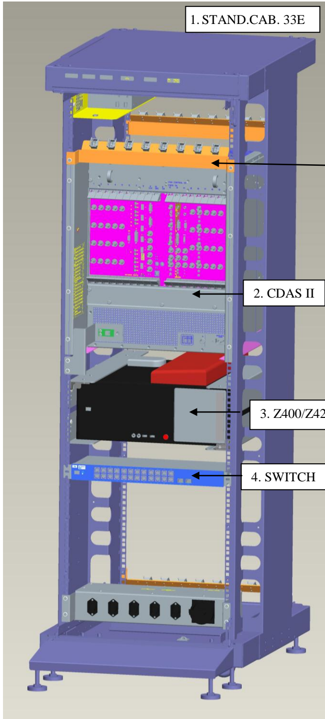
Figuur 1 Frontview NT-DAC
