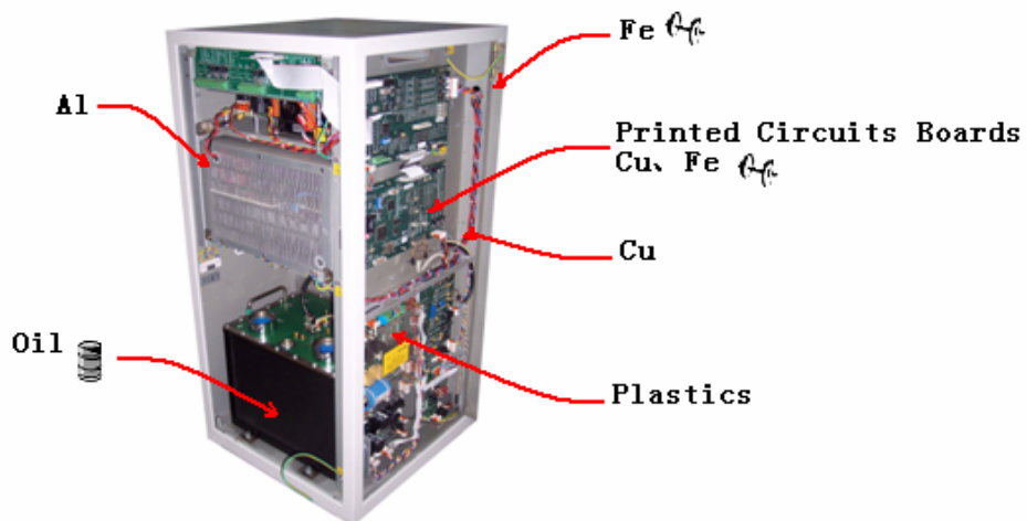
Fig 10 HV Generator
